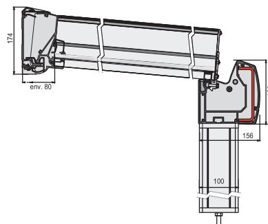
Essential : type affleurant B avec renfort acier
