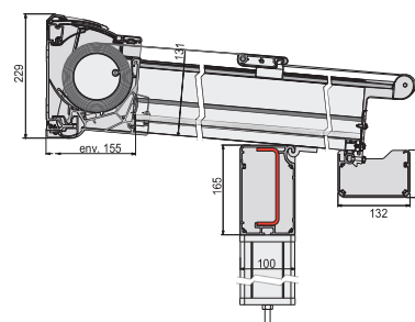
Integrale : type débordant Ü avec renfort acier
